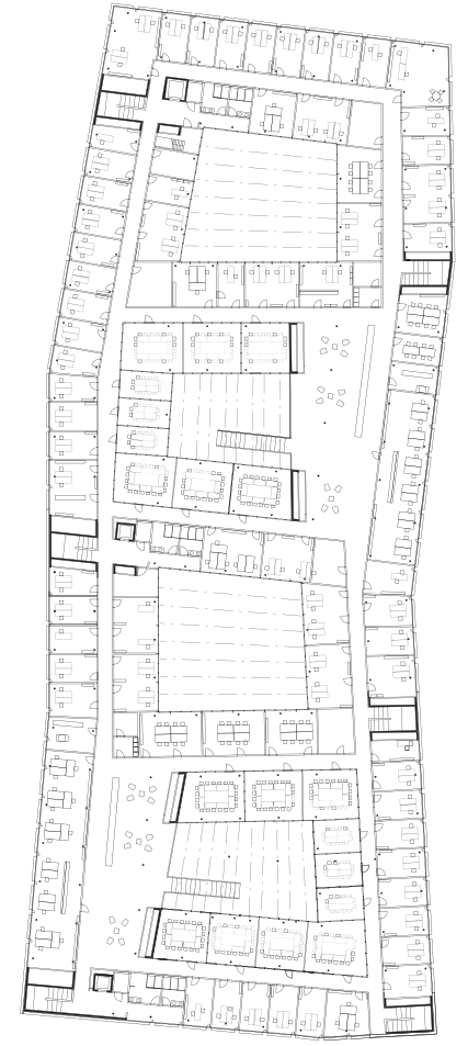
2. OBERGESCHOSS
