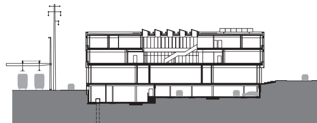
SCHNITT Kleiner Hof
