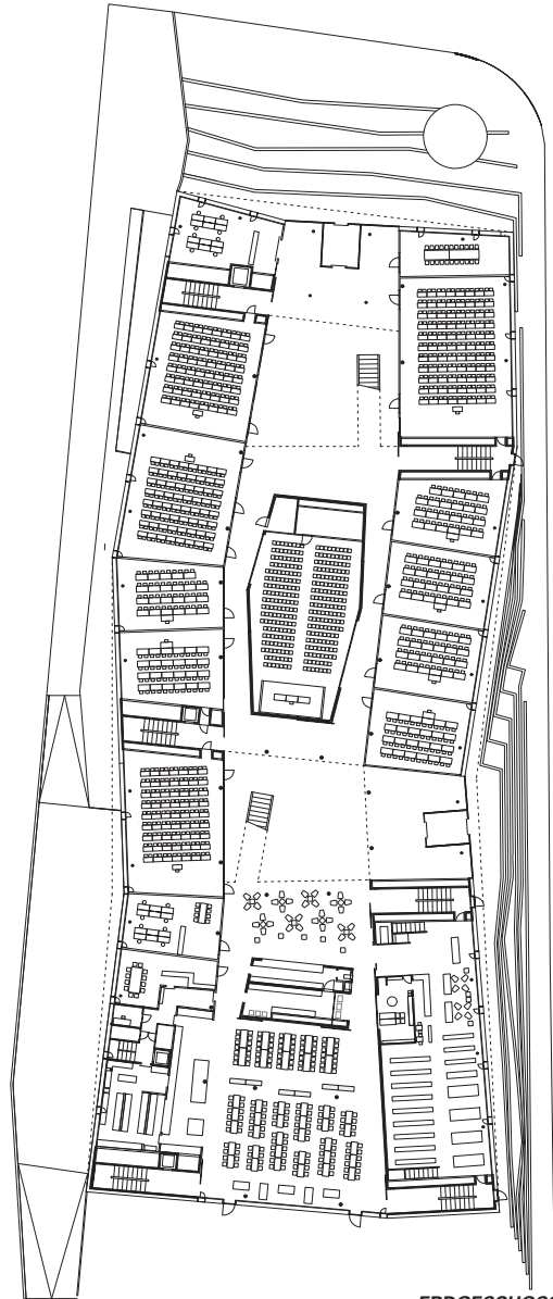
ERDGESCHOSS
